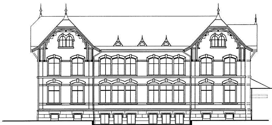
NORDFASSADE HAUS 13
